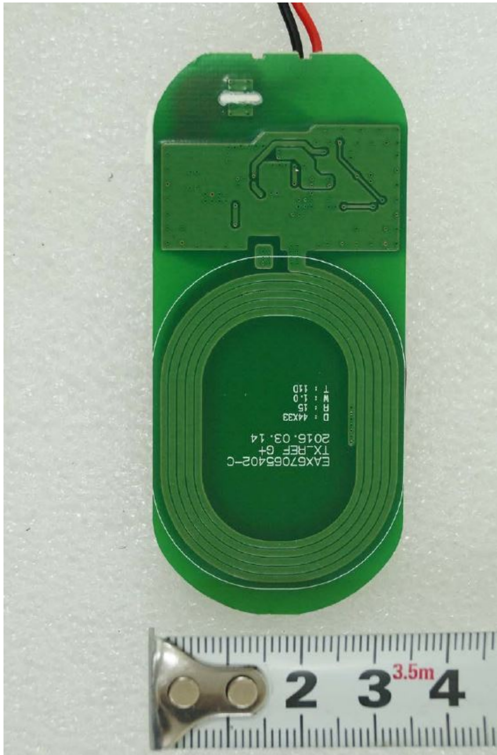
<Wireless shelf module -3>
