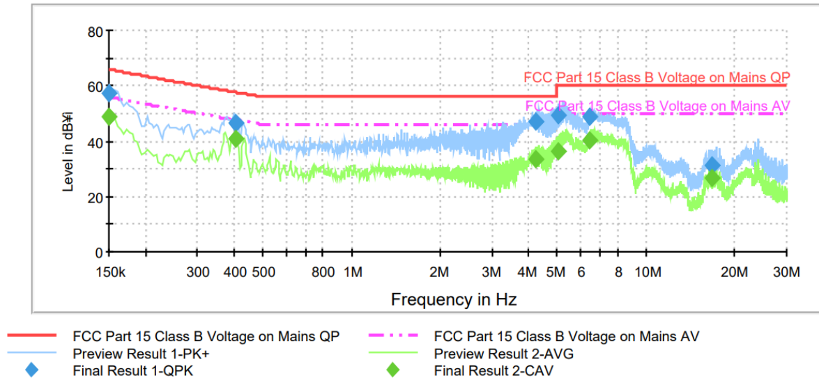
ESH2-Z5 150k-30M_2 LINE
