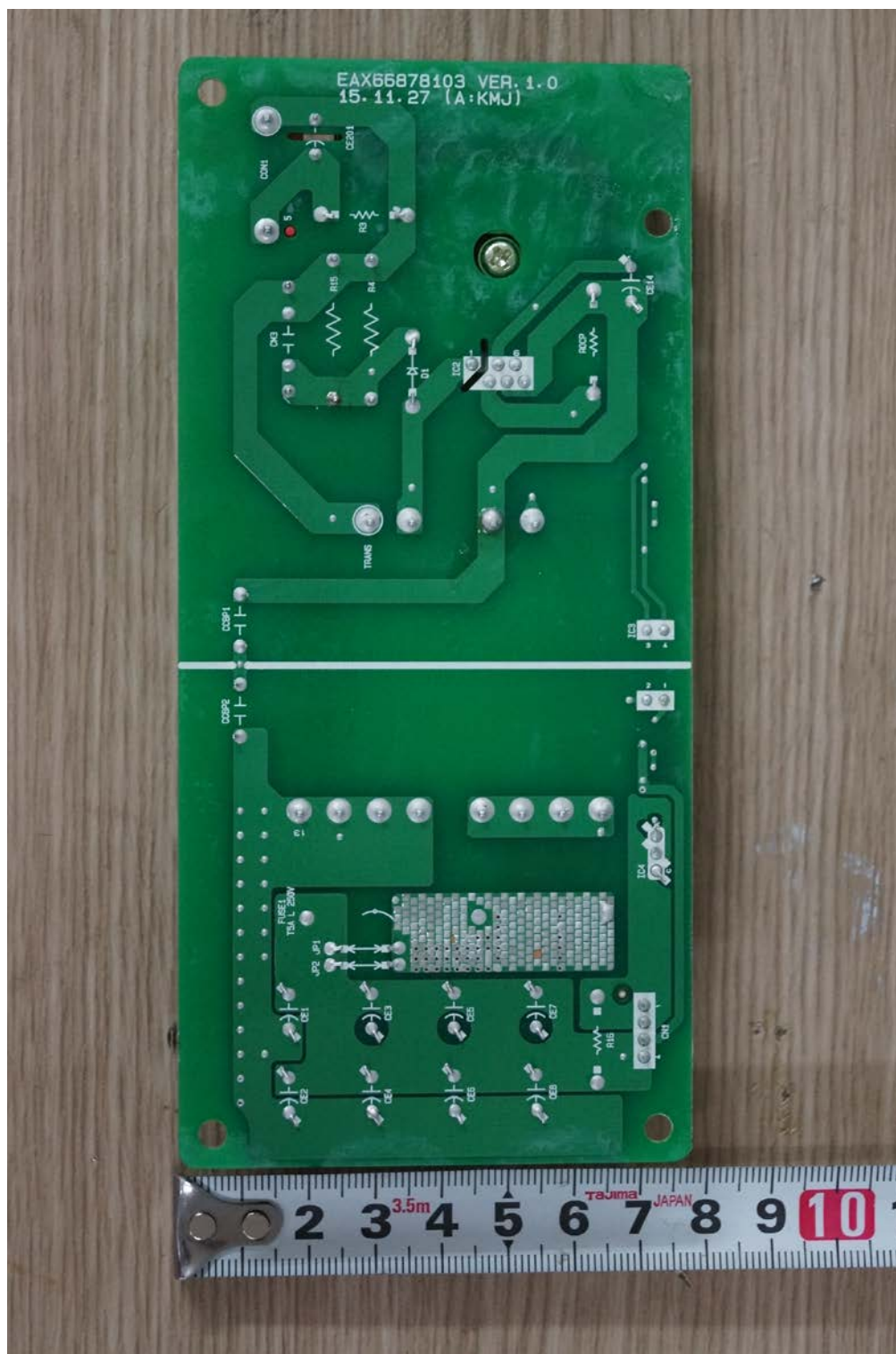
<Original Auto Door sub PCB>
