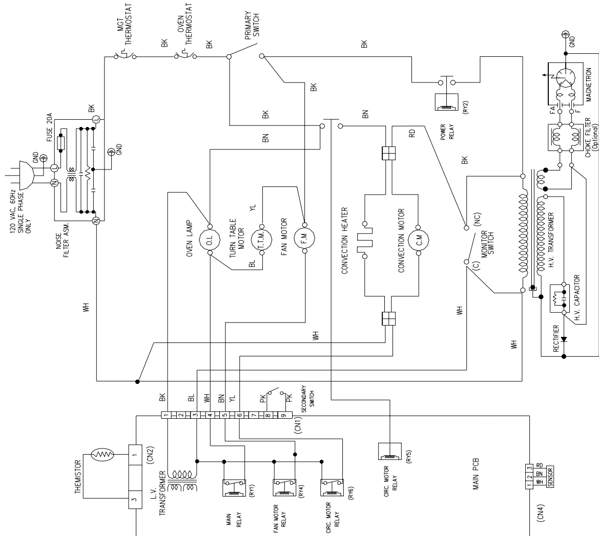
<Fig. 3. Schematic Diagram>
