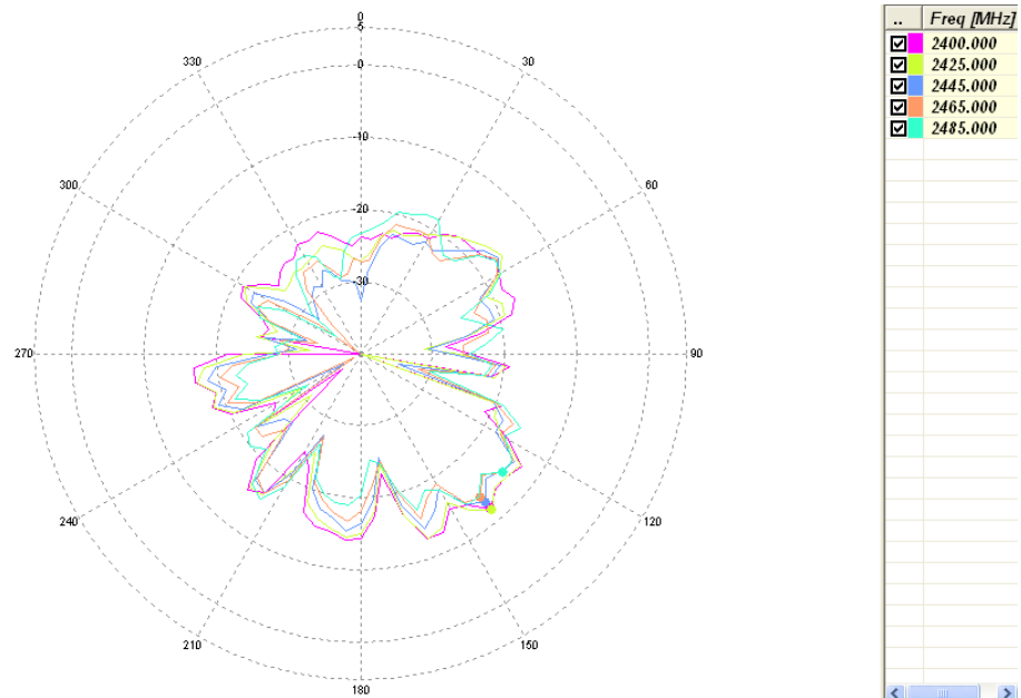
E2-Plan [Vertical]
