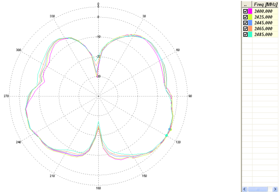
E1-Plan [Horizontal]
