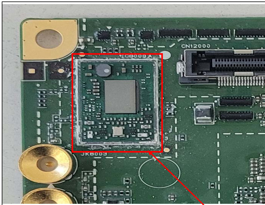
BT/WIFI Module
