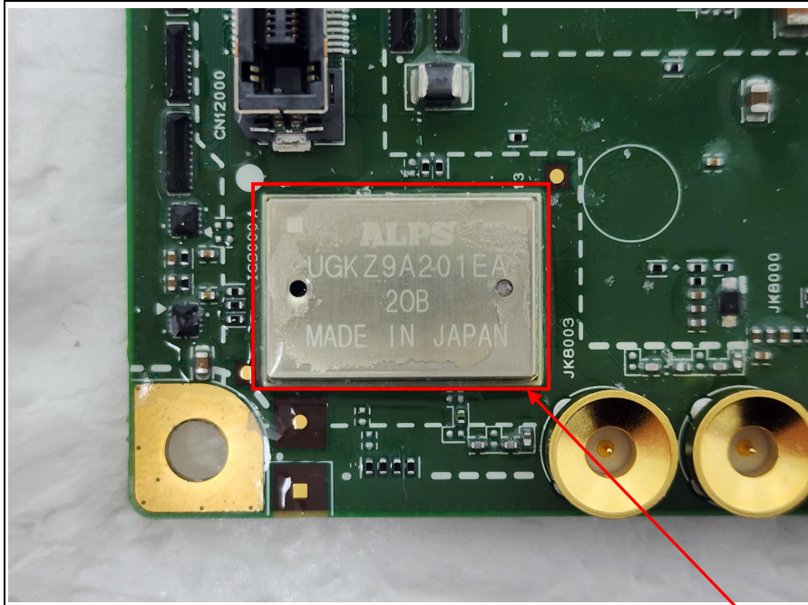
BT/WIFI Module
