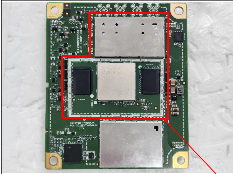
WWAN Module
