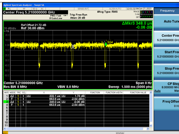
802.11ac(VHT80)
