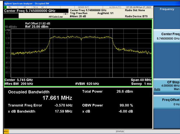
802.11ac(VHT20) (CH.149)
