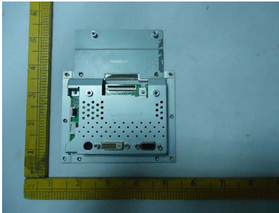
6) EUT Photo
