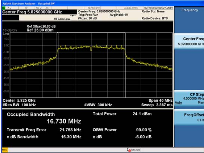
802.11a (CH.165)
