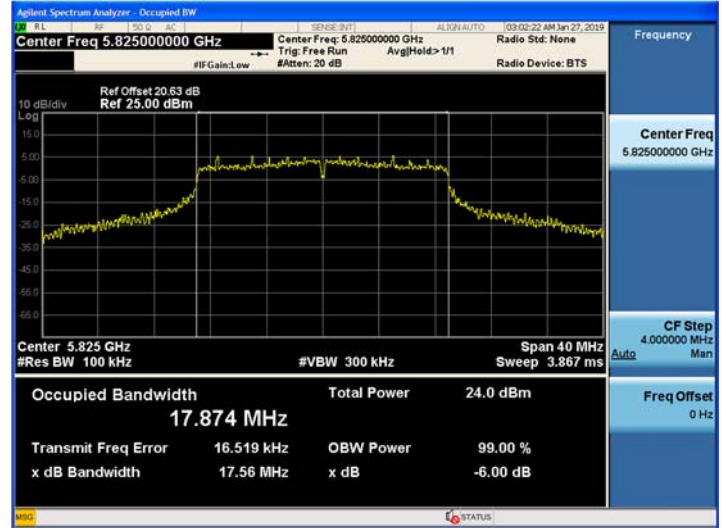
802.11n(HT20) (CH.165)
