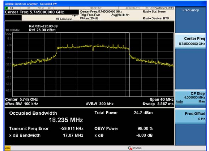
802.11n(HT20) (CH.149)
