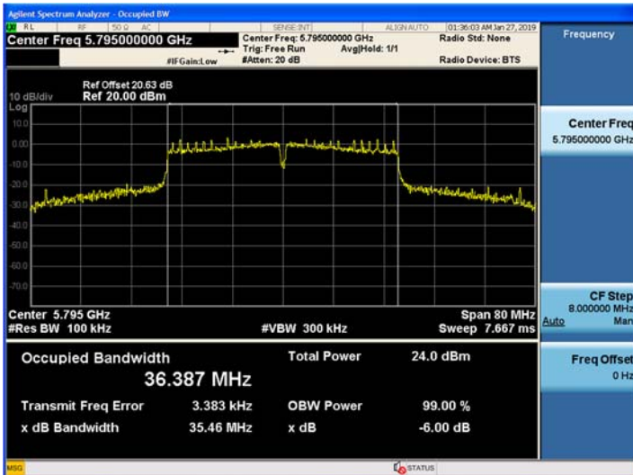
802.11n(HT40) (CH.159)
