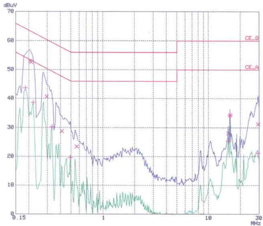
&lt; Hot line &gt;
