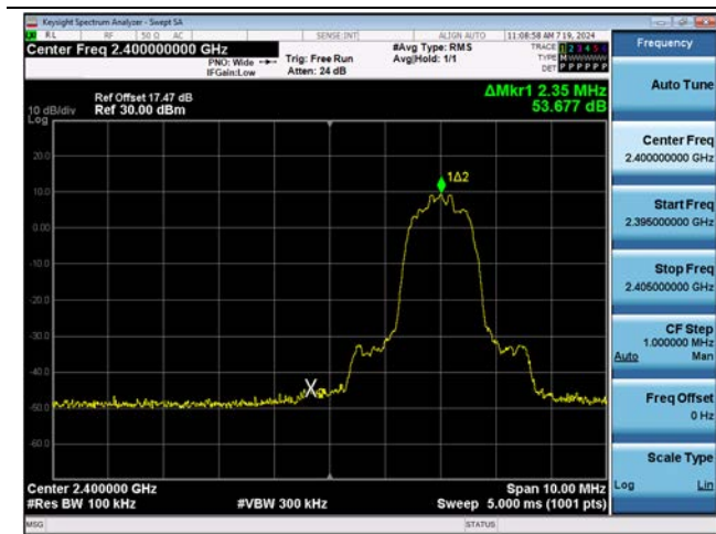
8DPSK Band Edge(CH.0)
