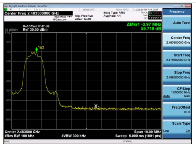
8DPSK Band Edge(CH.78)
