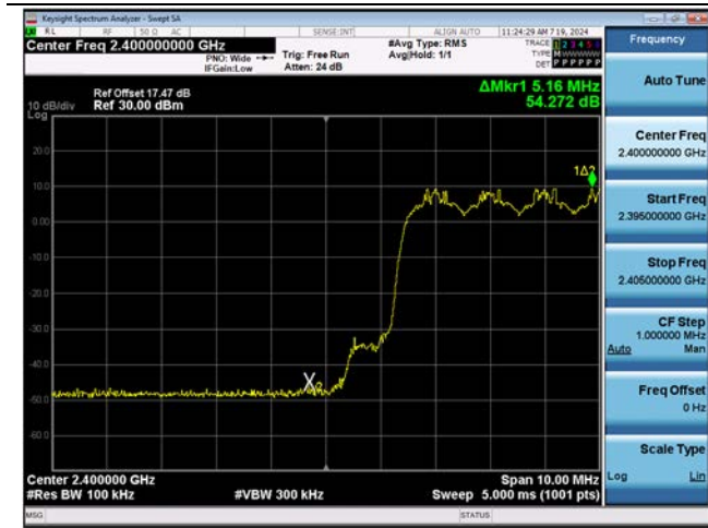
\pi/4 DQPSK Band Edge(CH.0)
