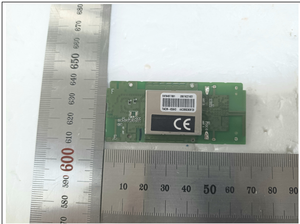
<WLAN Module>
