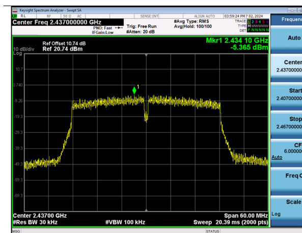
ANT. 1
