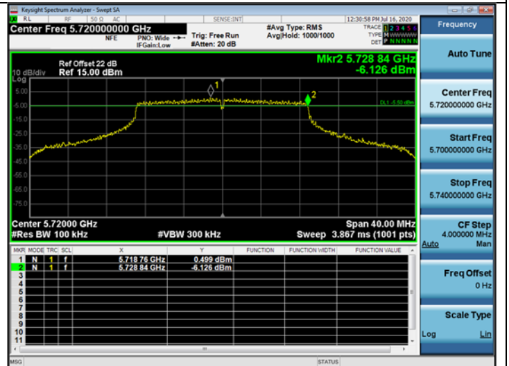
802.11n_HT20 CH.144
