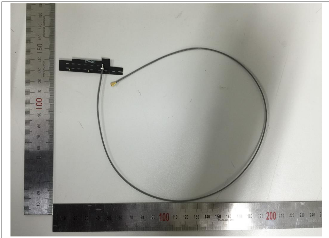
<Antenna 2>
