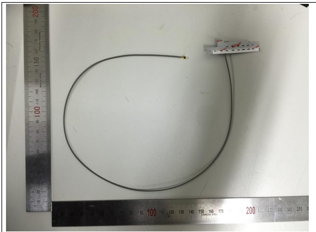
<Antenna 2>
