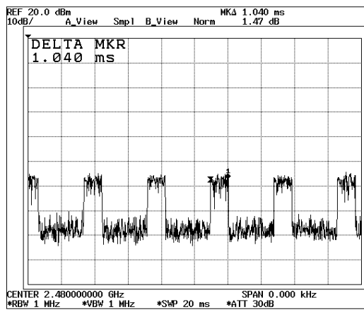
CH 78 2480MHz
