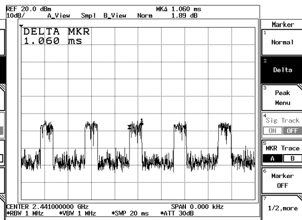
CH 39 2441MHz
