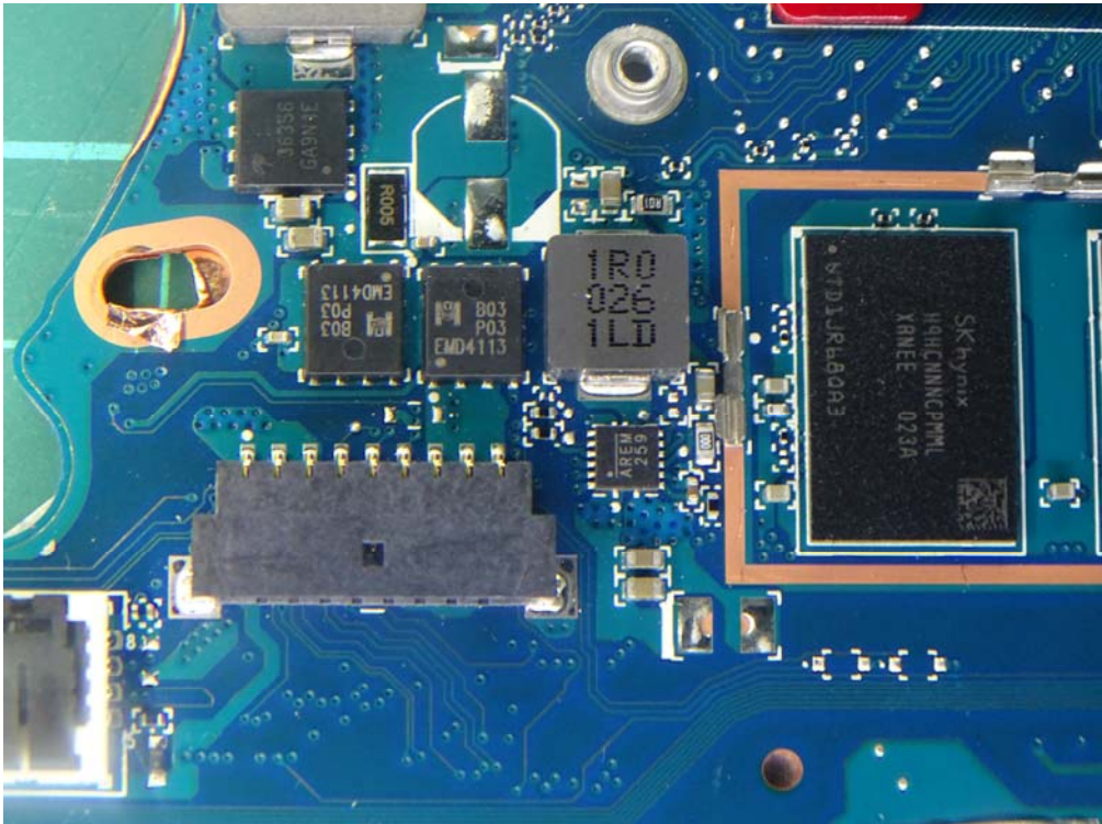
(44) EUT Photo
