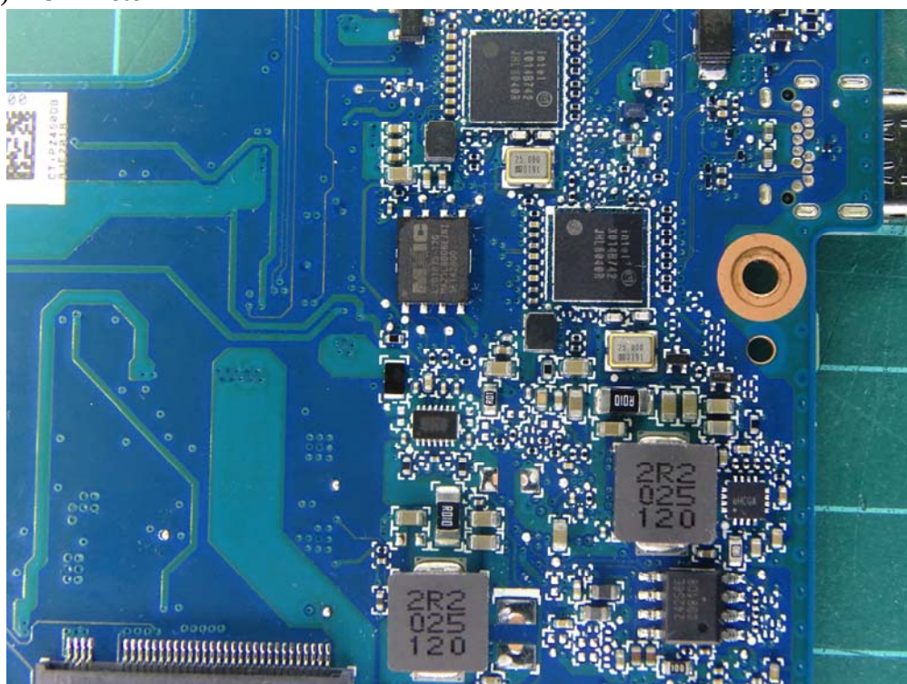
(47) EUT Photo
