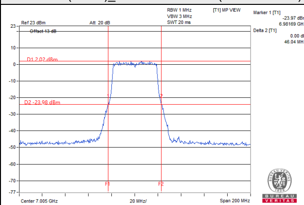
802.11ax (HE40)_Chain 1 / CH 211 (U-NII-8 Band)
