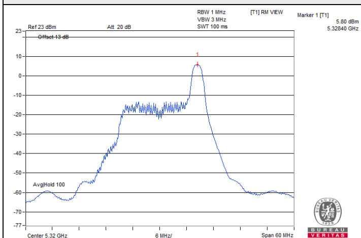
20 MHz Preamble 802.11ax (RU26) / Chain 1 : CH 64
