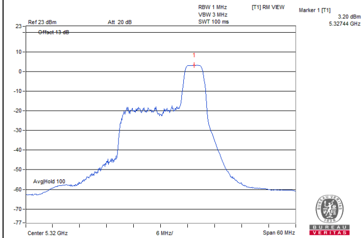
20 MHz Preamble 802.11ax (RU52) / Chain 1 : CH 64
