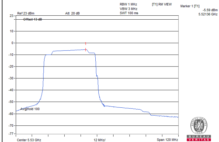
80 MHz Preamble 802.11ax (RU484) / Chain 0 : CH 106
