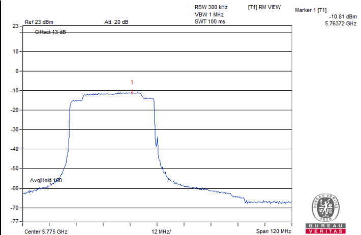
80 MHz Preamble 802.11ax (RU484) / Chain 0 : CH 155
