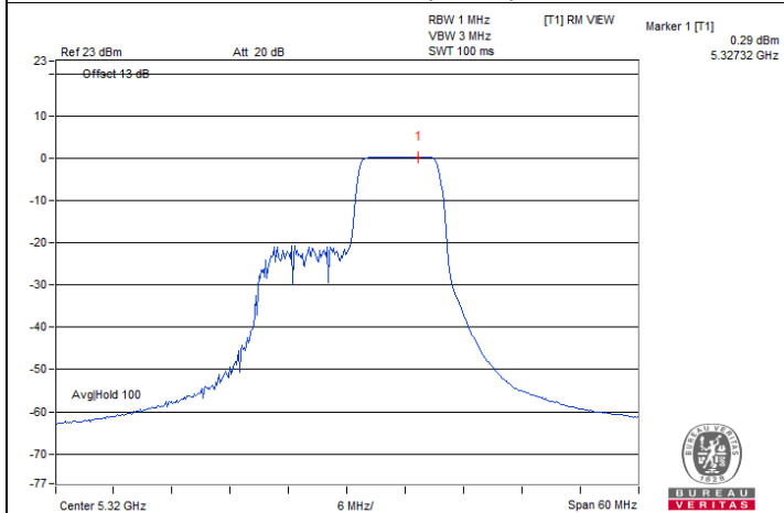
20 MHz Preamble 802.11ax (RU106) / Chain 1 : CH 64
