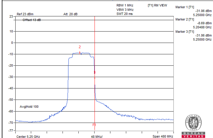
160 MHz Preamble 802.11ax (RU996) / Chain 1 : CH 50 (U-NII-1)
