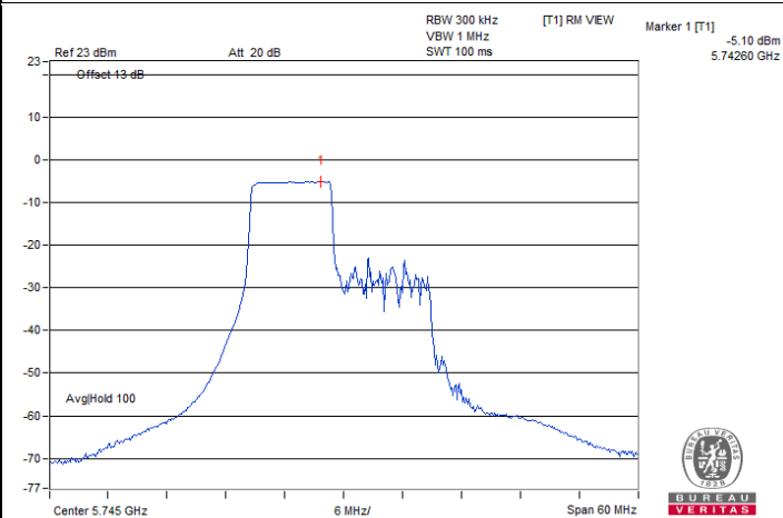
20 MHz Preamble 802.11ax (RU106) / Chain 1 : CH 149
