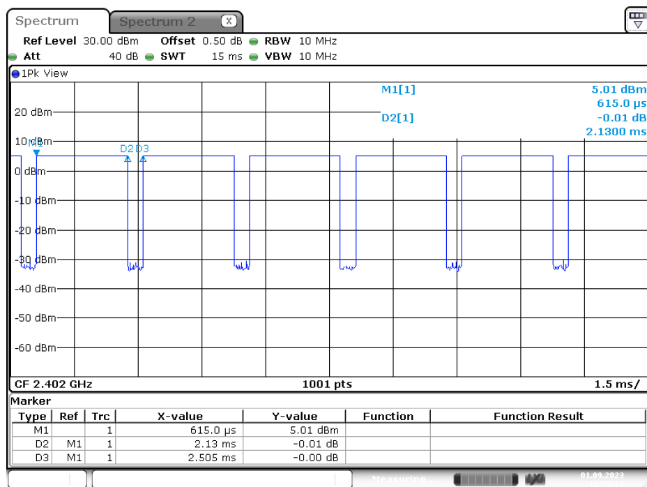
BLE 1M
