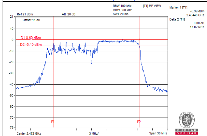
20 MHz Preamble 802.11ax (RU106) / Chain 1 : CH 13
