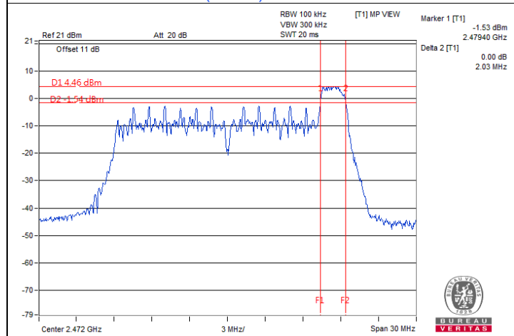
20 MHz Preamble 802.11ax (RU26) / Chain 0 : CH 13
