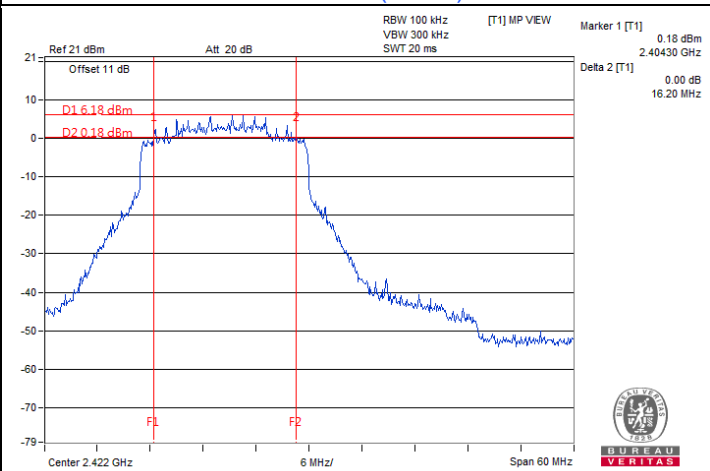
40 MHz Preamble 802.11ax (RU242) / Chain 0 : CH 3
