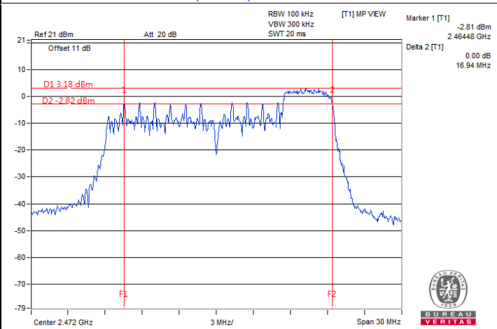
20 MHz Preamble 802.11ax (RU52) / Chain 0 : CH 13
