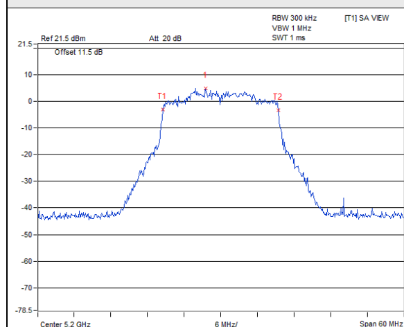
802.11ax (HE20) / Chain 0 : CH 40
