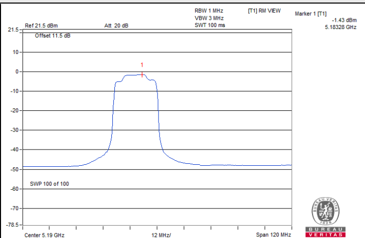
40 MHz Preamble 802.11ax (RU242) / Chain 1 : CH 38
