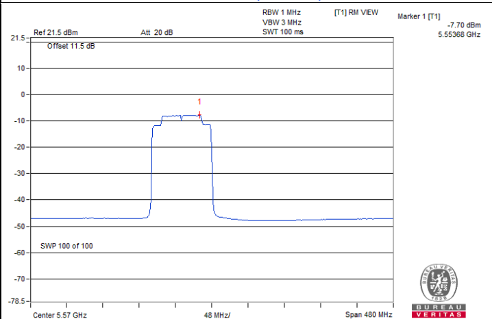
160 MHz Preamble 802.11ax (RU996) / Chain 1 : CH 114
