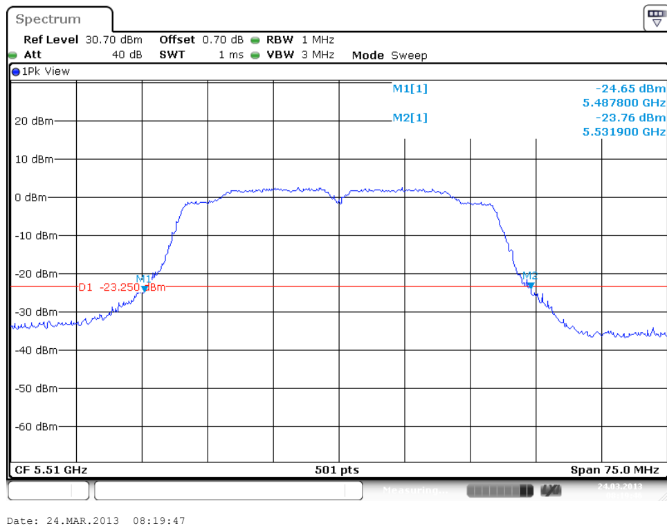
Plot A2 Antenna 2
