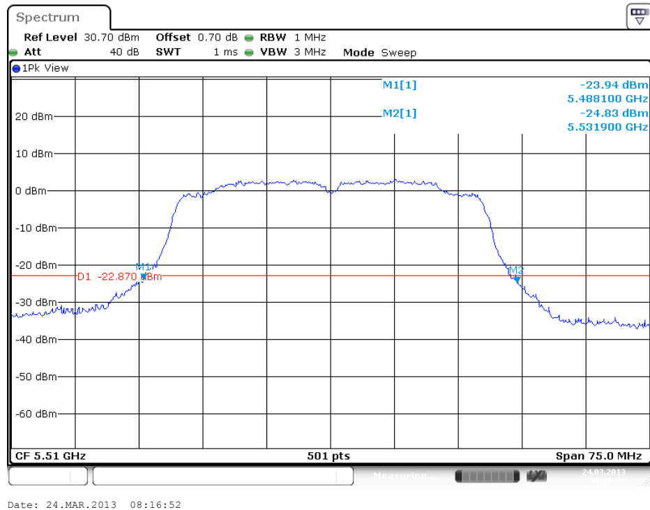
Plot A1 Antenna 1
