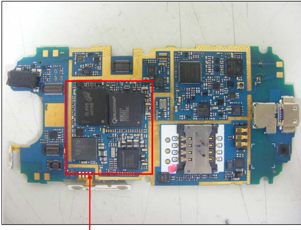
BT & WLAN module
