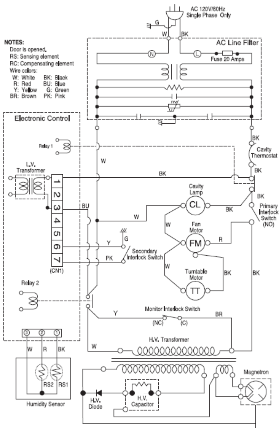
<Fig. 3. Schematic Diagram>
