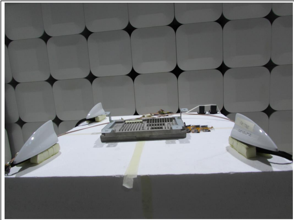
EUT Position: X-axis #2
