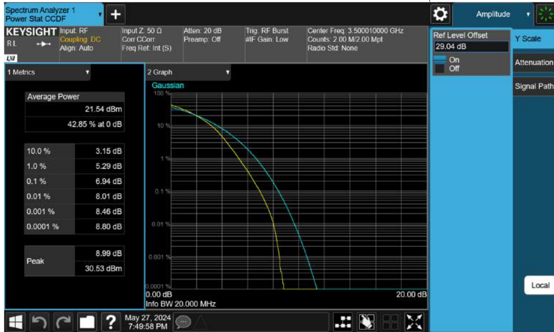
Sub6 n77(78). PAR Plot (20 M BW_Ch.633334_256 QAM)
