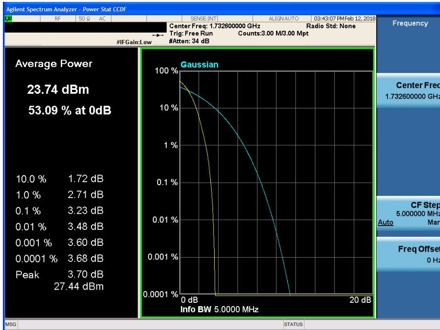
WCDMA1700 & Channel: 1413
