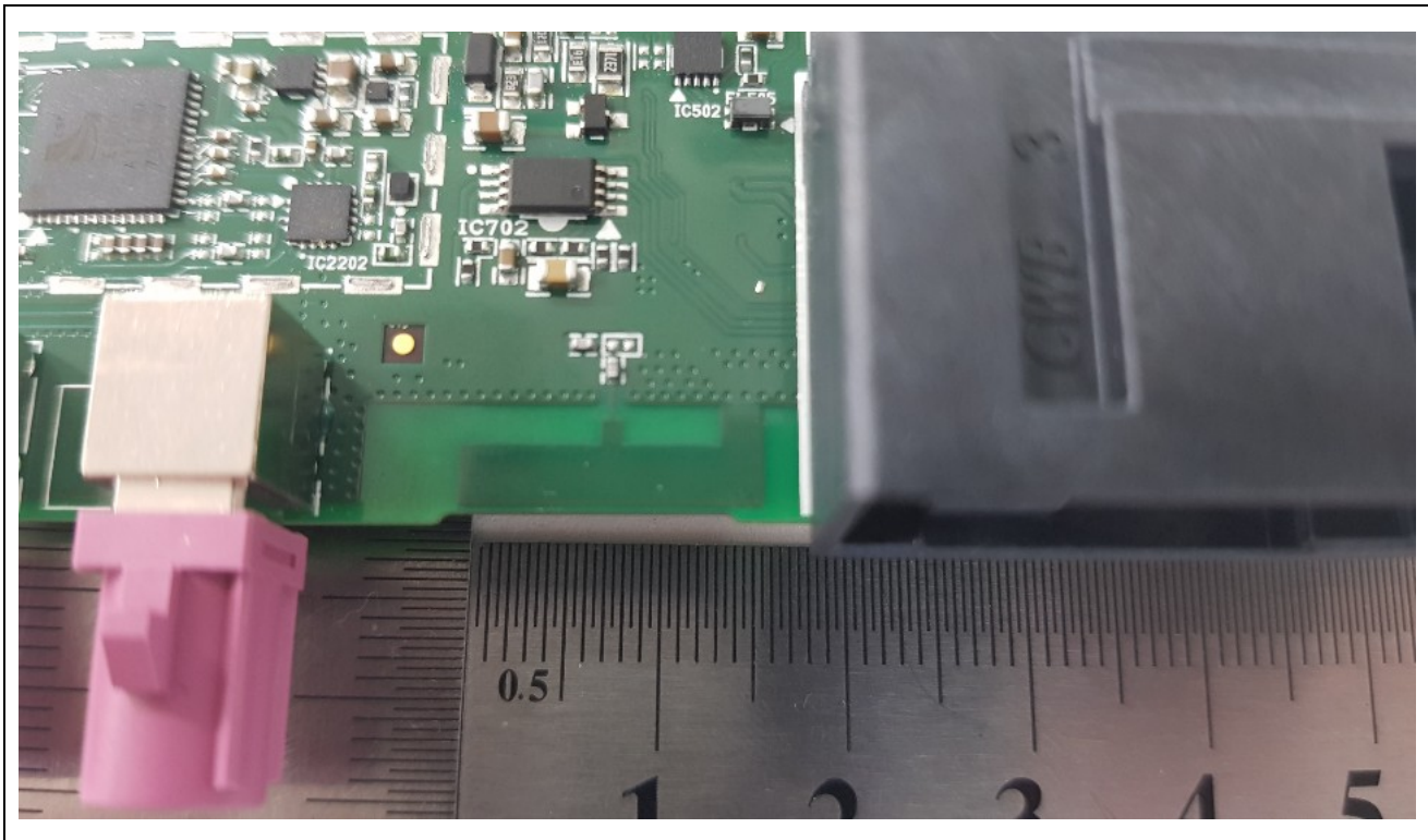
<WLAN Antenna>
