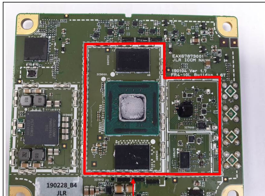
WWAN Module
