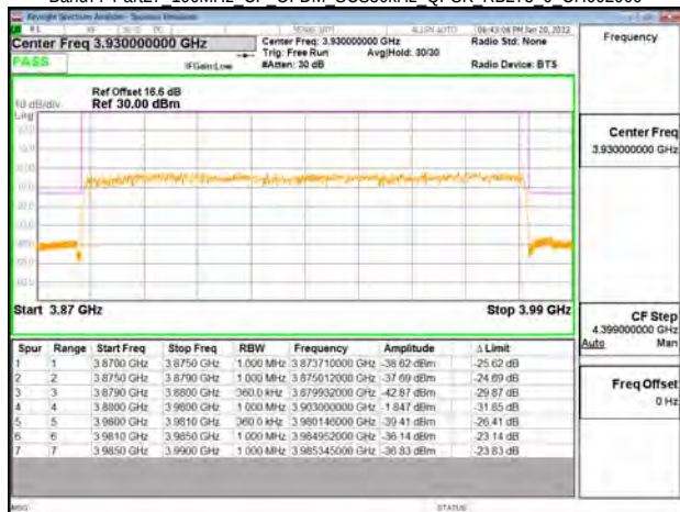
Band77-Part27 100MHz CP OFDM SCS30kHz QPSK RB273 0 CH662000
