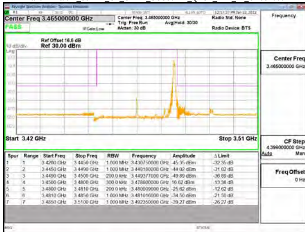
Band77-Part27 30MHz CP OFDM SCS30kHz QPSK RB1 77 CH633334
