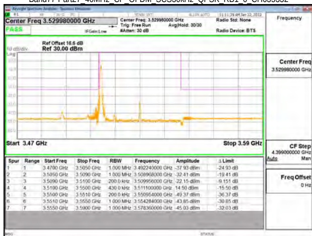
Band77-Part27 40MHz CP OFDM SCS30kHz QPSK RB1 0 CH635332
