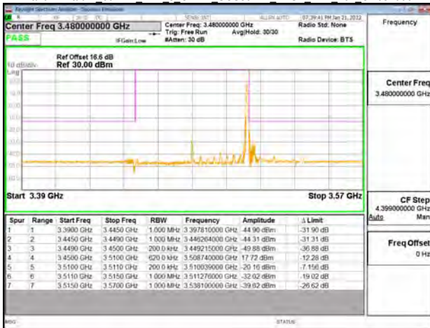
Band77-Part27 60MHz DFT s OFDM SCS30kHz BPSK RB1 161 CH633334
