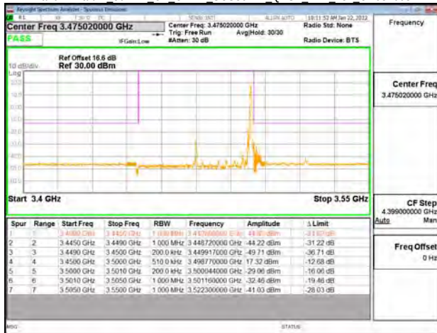
Band77-Part27 50MHz CP OFDM SCS30kHz QPSK RB1 132 CH633334
