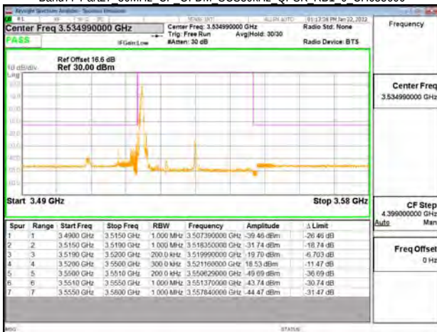
Band77-Part27 30MHz CP OFDM SCS30kHz QPSK RB1 0 CH635666
