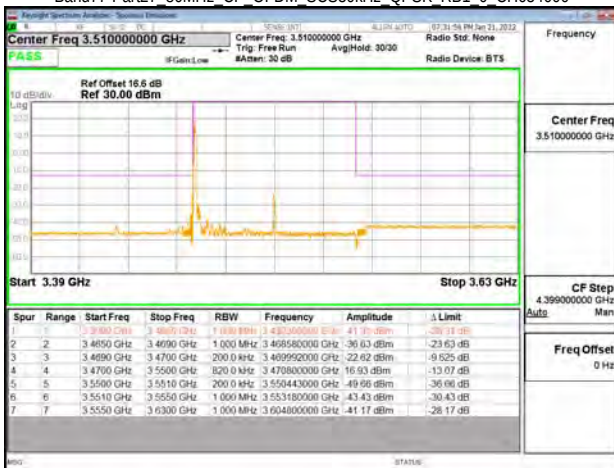
Band77-Part27 80MHz CP OFDM SCS30kHz QPSK RB1 0 CH634000
