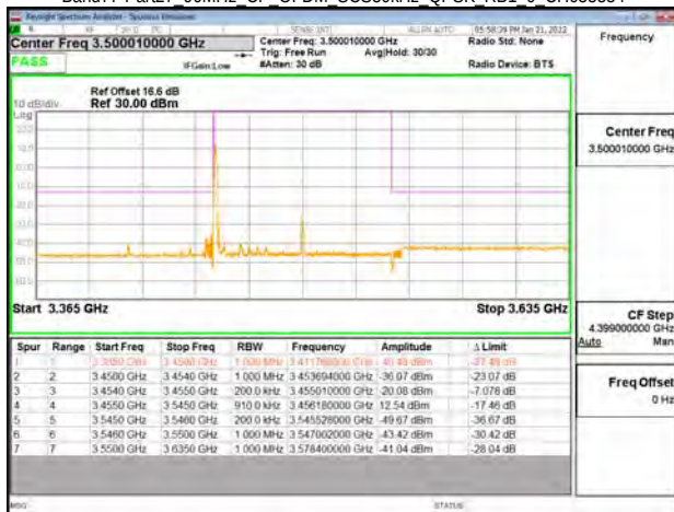
Band77-Part27 90MHz CP OFDM SCS30kHz QPSK RB1 0 CH633334
