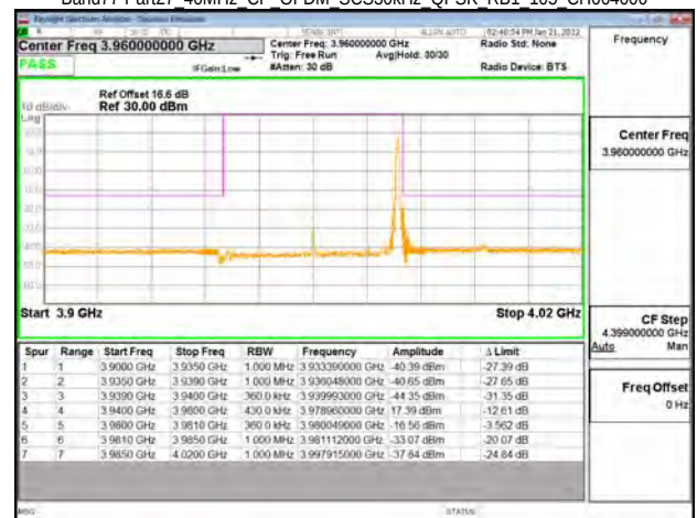
Band77-Part27 40MHz CP OFDM SCS30kHz QPSK RB1 105 CH664000
