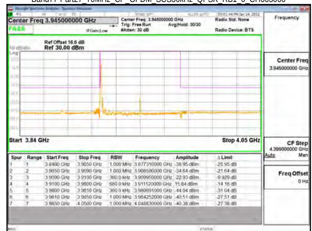
Band77-Part27 70MHz CP OFDM SCS30kHz QPSK RB1 0 CH663000
