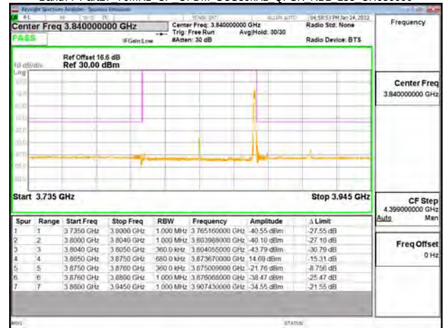
Band77-Part27 70MHz CP OFDM SCS30kHz QPSK RB1 188 CH663000
