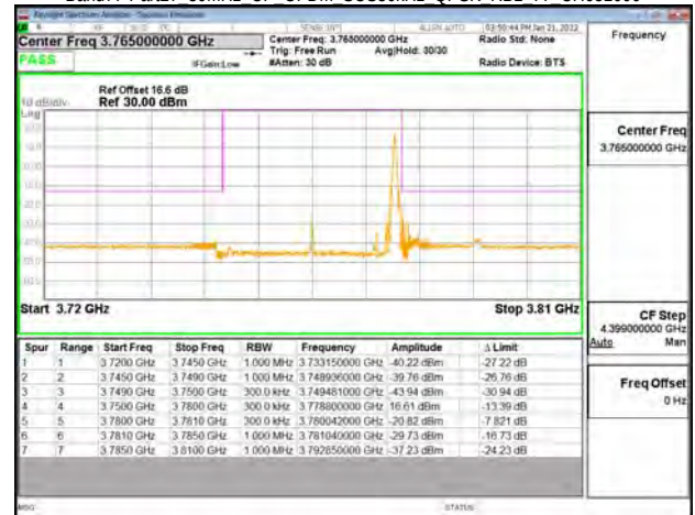
Band77-Part27 30MHz CP OFDM SCS30kHz QPSK RB1 77 CH656000
