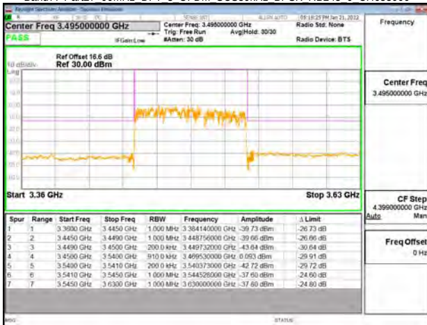
Band77-Part27 90MHz DFT s OFDM SCS30kHz BPSK RB243 0 CH633334
