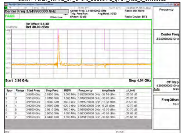
Band77-Part27 60MHz CP OFDM SCS30kHz QPSK RB1 0 CH663332
