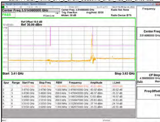
Band77-Part27 70MHz DFT s OFDM SCS30kHz BPSK RB1 188 CH634332
