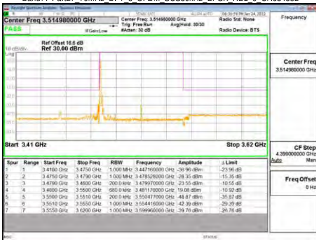
Band77-Part27 70MHz DFT s OFDM SCS30kHz BPSK RB1 0 CH634332
