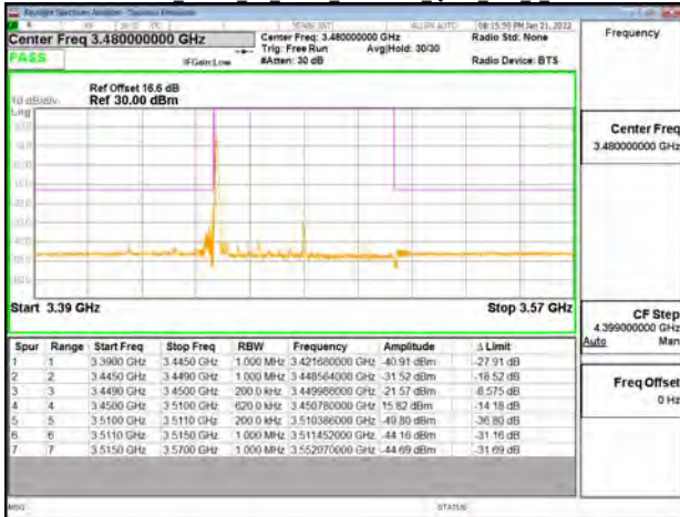
Band77-Part27 60MHz CP OFDM SCS30kHz QPSK RB1 0 CH633334
