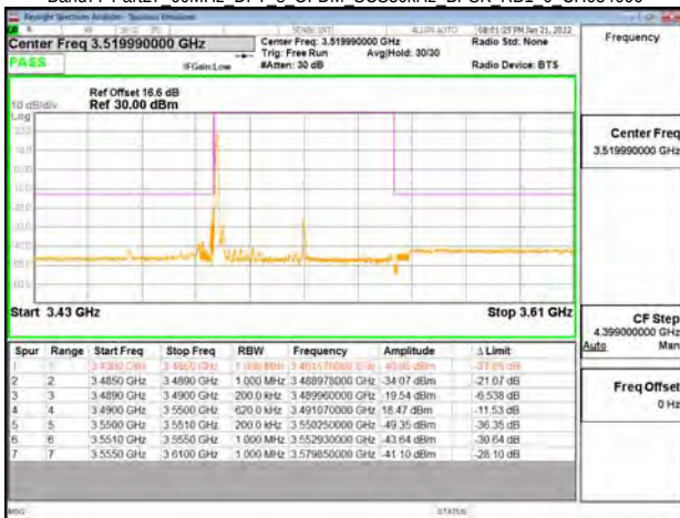
Band77-Part27 60MHz DFT s OFDM SCS30kHz BPSK RB1 0 CH634666
