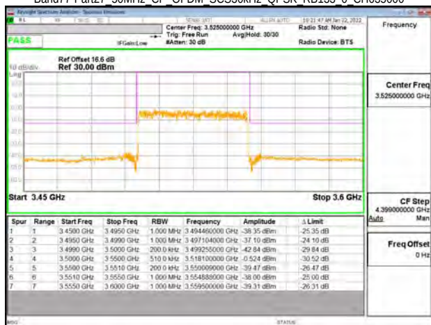
Band77-Part27 50MHz CP OFDM SCS30kHz QPSK RB133 0 CH635000
