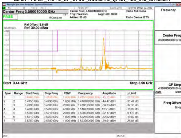
Band77-Part27 40MHz CP OFDM SCS30kHz QPSK RB1 105 CH635332
