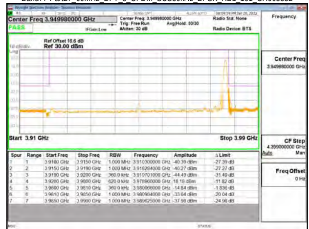
Band77-Part27 60MHz DFT s OFDM SCS30kHz BPSK RB1 161 CH633332
