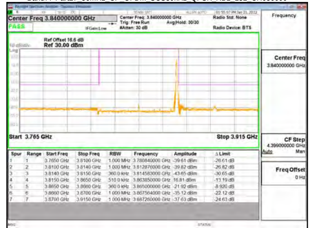
Band77-Part27 50MHz CP OFDM SCS30kHz QPSK RB1 132 CH663666
