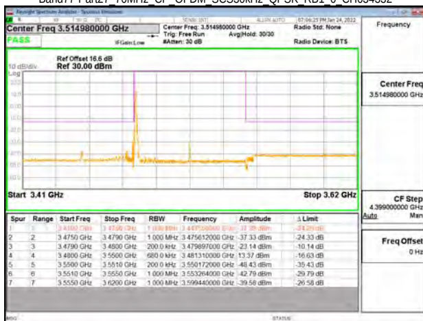
Band77-Part27 70MHz CP OFDM SCS30kHz QPSK RB1 0 CH634332
