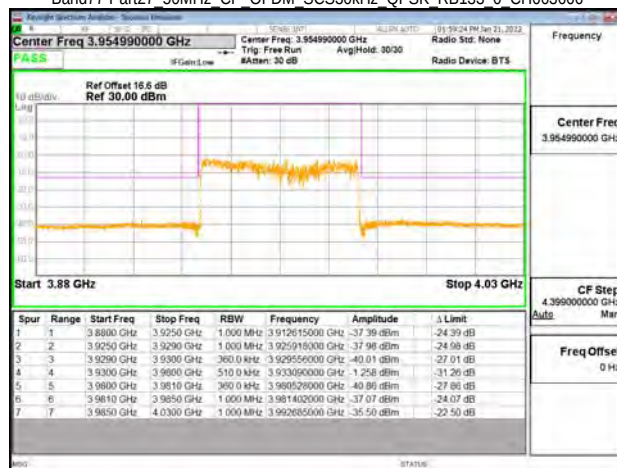
Band77-Part27 50MHz CP OFDM SCS30kHz QPSK RB133 0 CH663666
