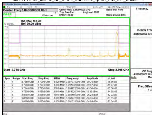
Band77-Part27 90MHz CP OFDM SCS30kHz QPSK RB1 244 CH656000
