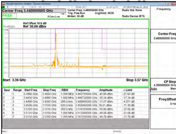
Band77-Part27 60MHz DFT s OFDM SCS30kHz BPSK RB1 0 CH633334
