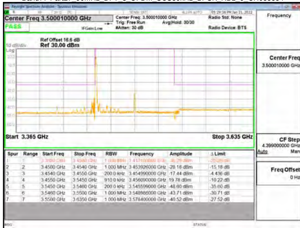
Band77-Part27 90MHz DFT s OFDM SCS30kHz BPSK RB1 0 CH633666
