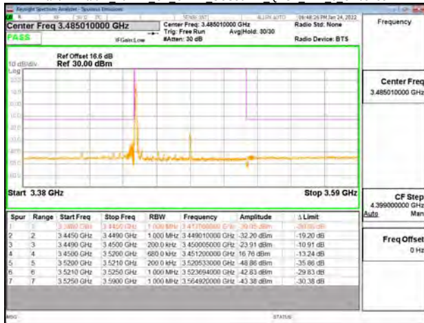
Band77-Part27 70MHz CP OFDM SCS30kHz QPSK RB1 0 CH633334
