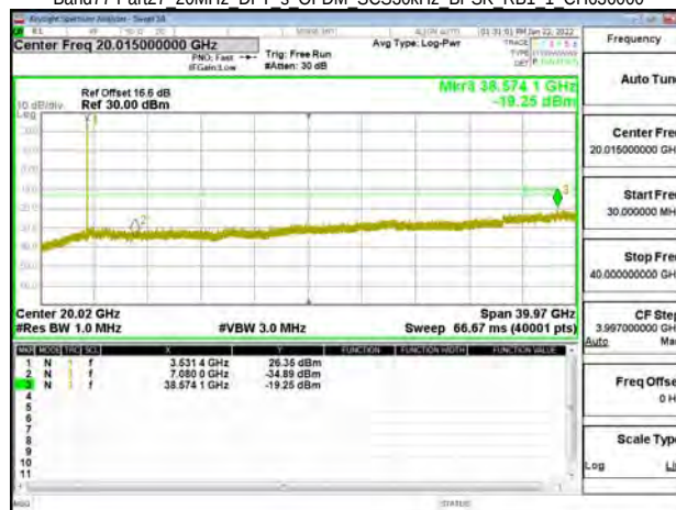
Band77-Part27 20MHz DFT s OFDM SCS30kHz BPSK RB1 1 CH630600
