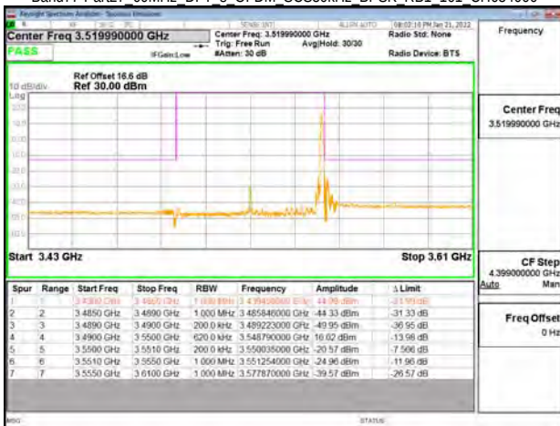
Band77-Part27 60MHz DFT s OFDM SCS30kHz BPSK RB1 161 CH634666
