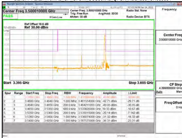
Band77-Part27 70MHz CP OFDM SCS30kHz QPSK RB1 188 CH634332
