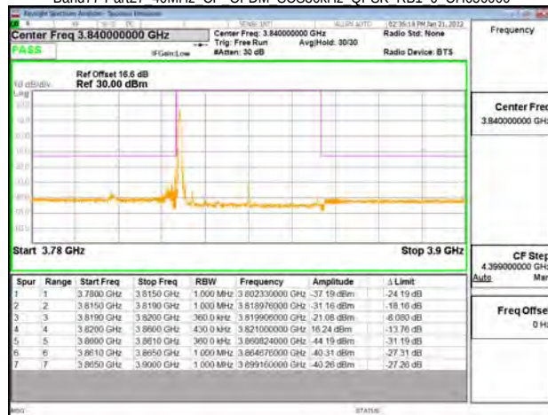
Band77-Part27 40MHz CP OFDM SCS30kHz QPSK RB1 0 CH646000
