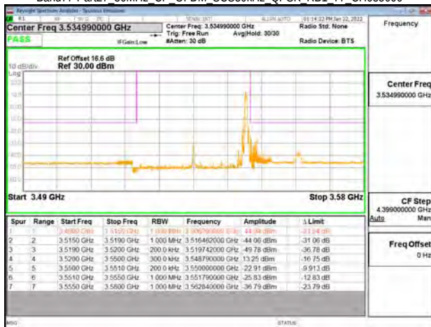
Band77-Part27 30MHz CP OFDM SCS30kHz QPSK RB1 77 CH635666
