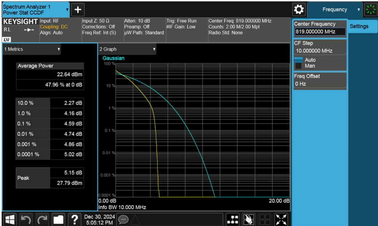
Sub6 n26. PAR Plot (10 M BW Ch.163800 QPSK RB 50_0)
