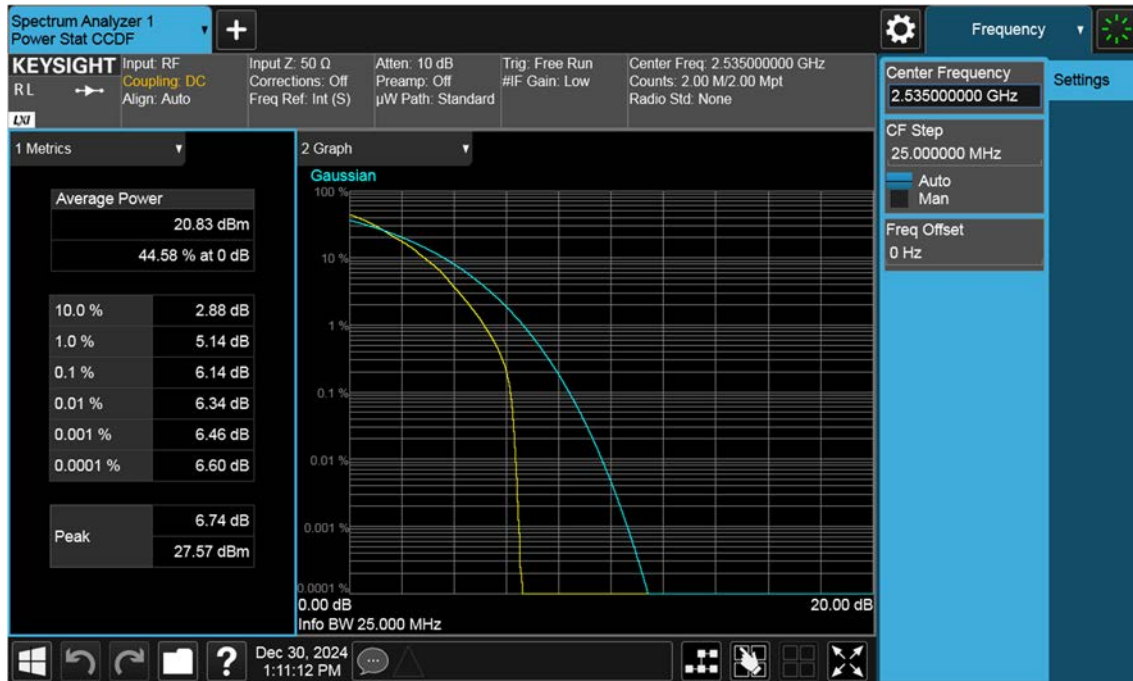
Sub6 n7. PAR Plot (25 M BW_Ch.507000_64QAM)
