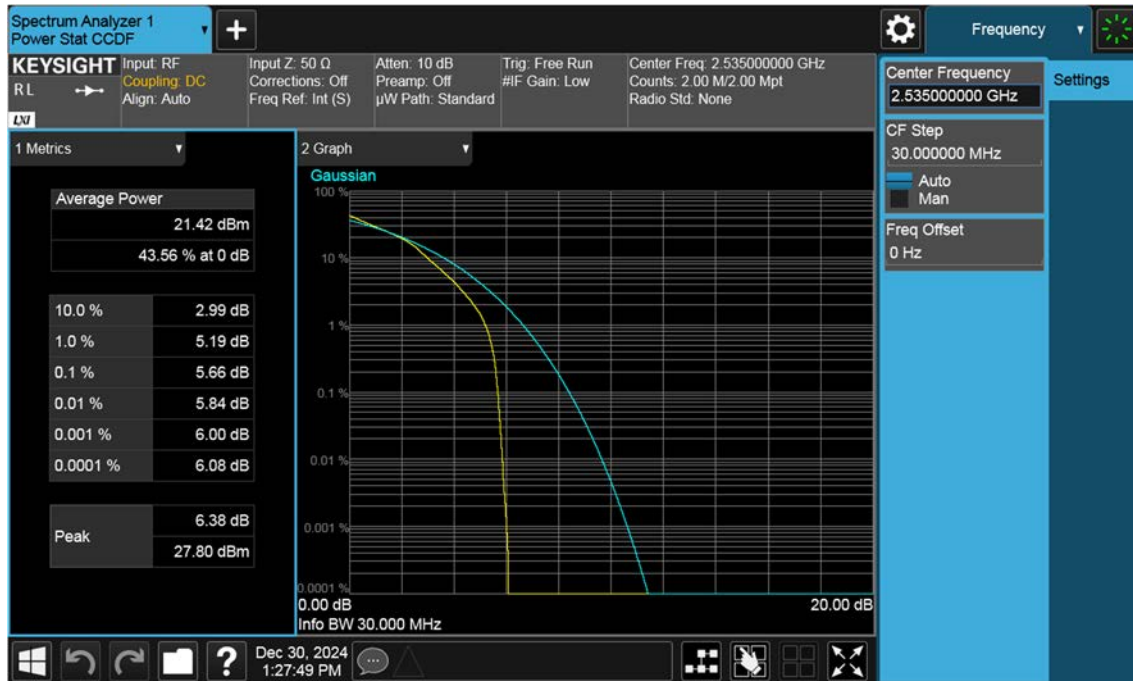
Sub6 n7. PAR Plot (30 M BW_Ch.507000_16QAM)
