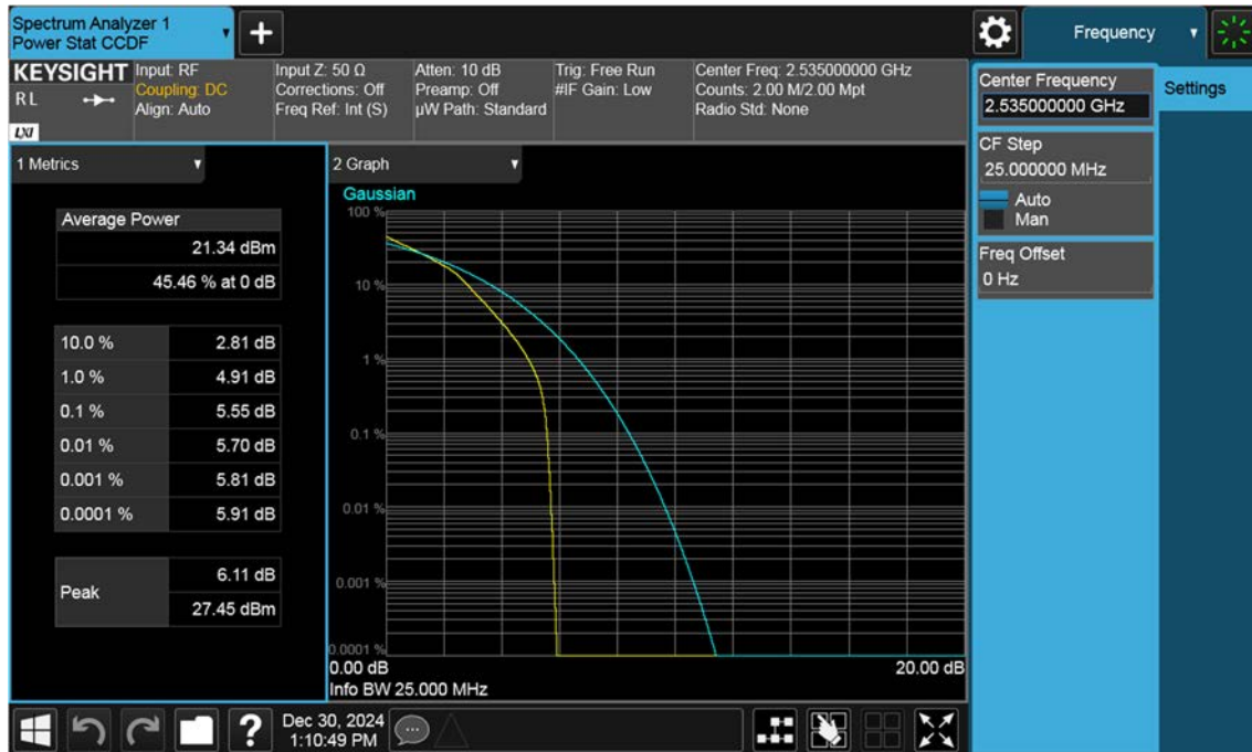
Sub6 n7. PAR Plot (25 M BW_Ch.507000_16QAM)
