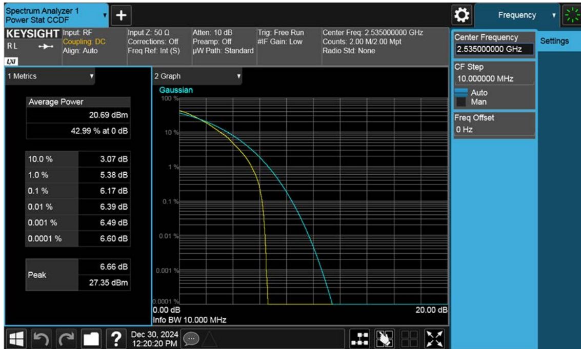
Sub6 n7. PAR Plot (10 M BW_Ch.507000_64QAM)
