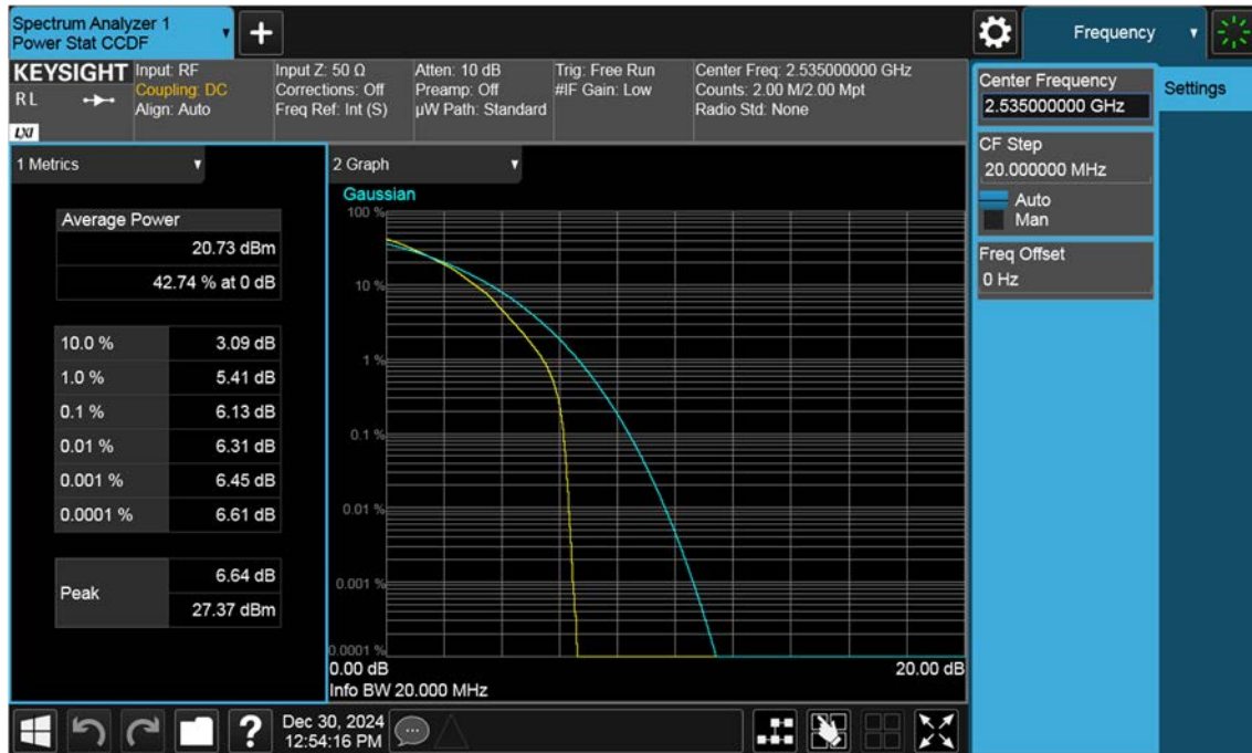
Sub6 n7. PAR Plot (20 M BW_Ch.507000_64QAM)
