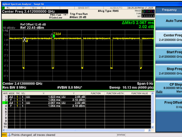
802.11n(HT20) (MCS0)
