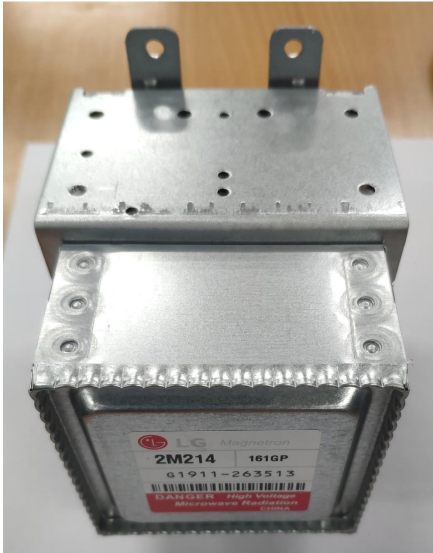
Magnetron: Model: 2M214
