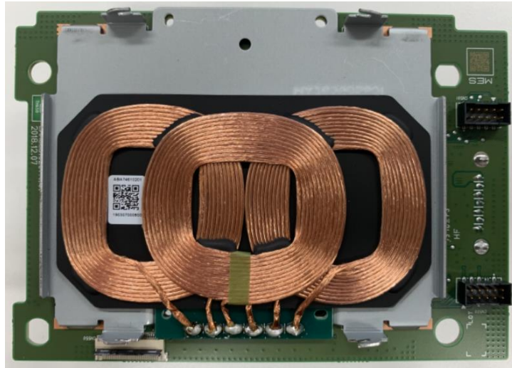
PCBA TOP
