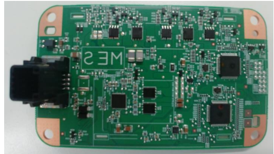
PCBA BOTTOM
