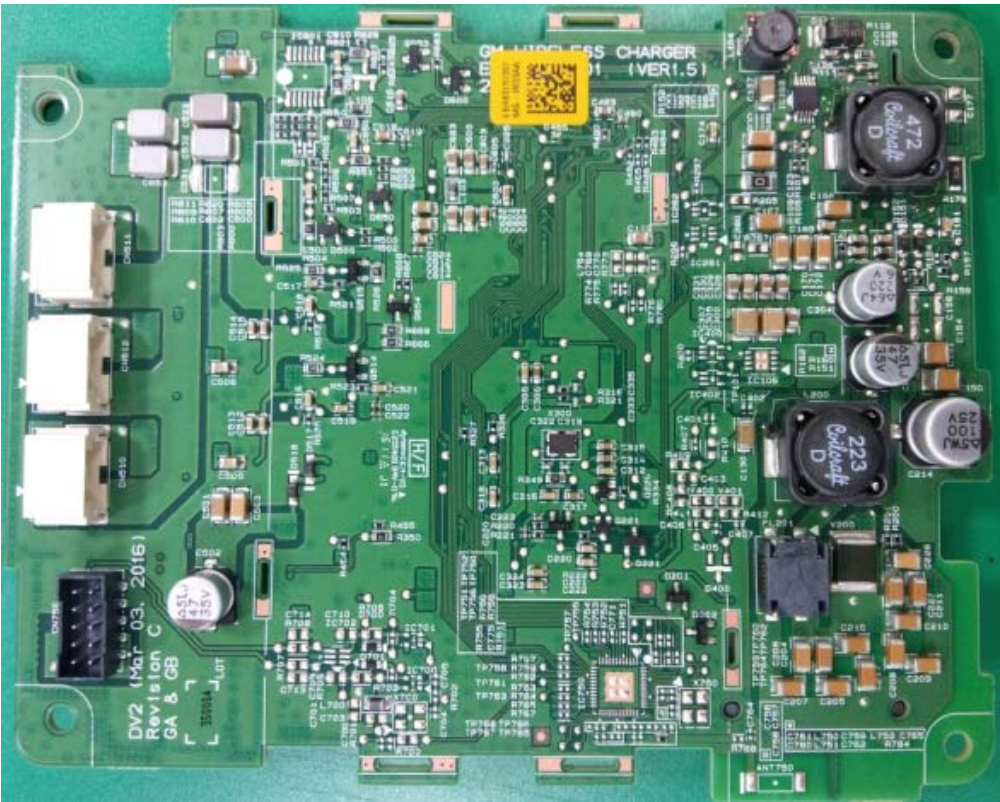
PCBA TOP
