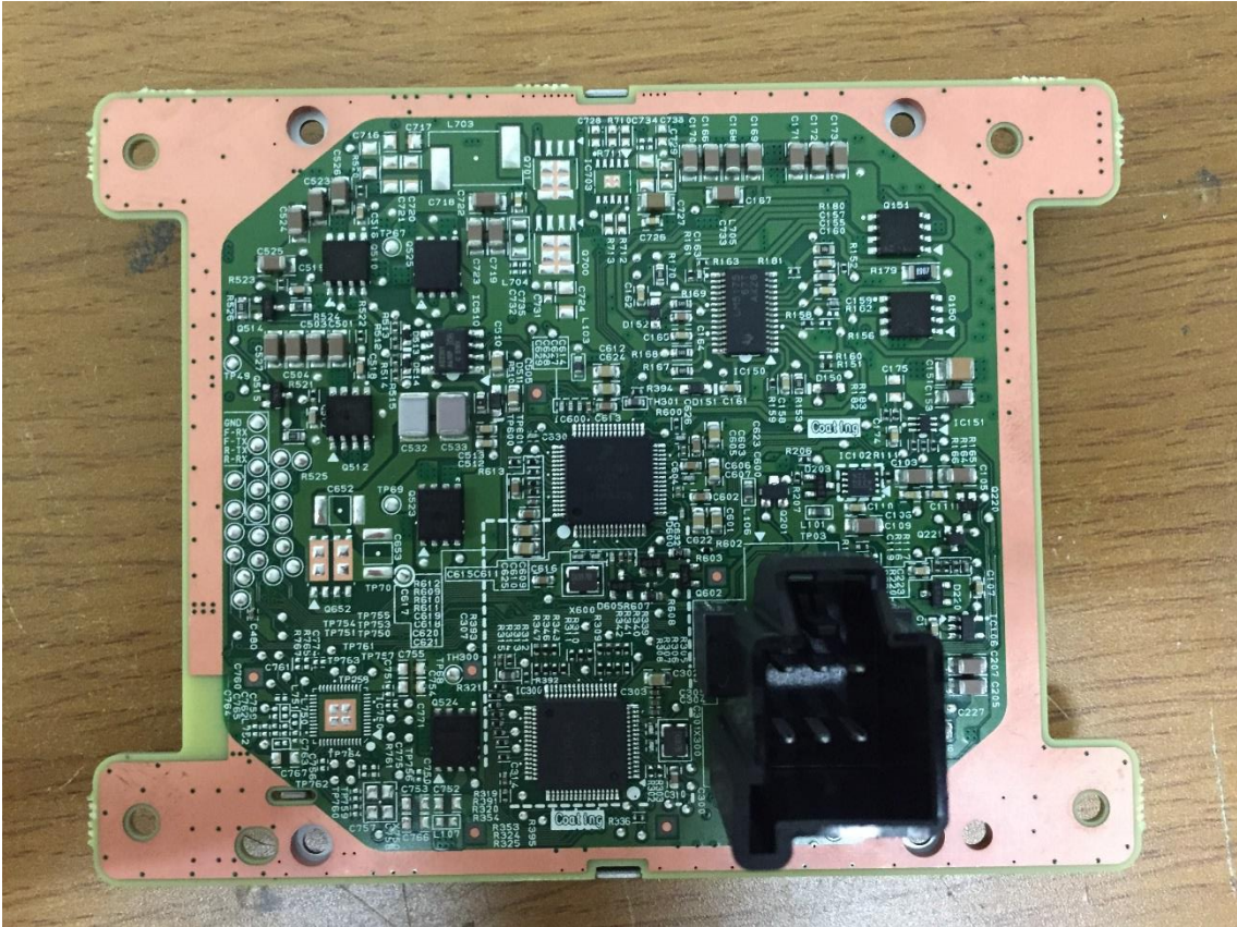
PCB BOTTOM
