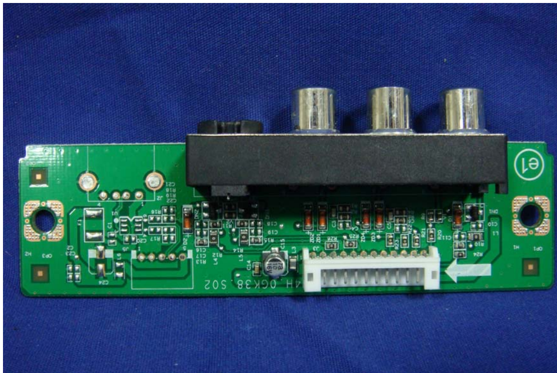
(17) EUT Photo
