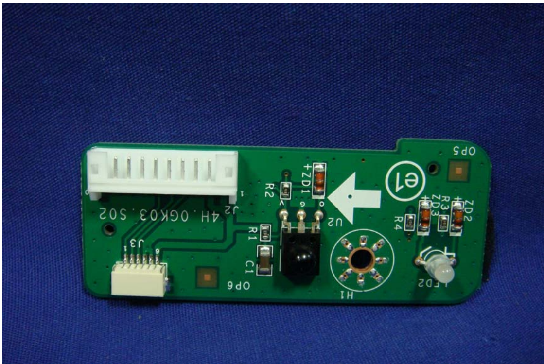
(19) EUT Photo
