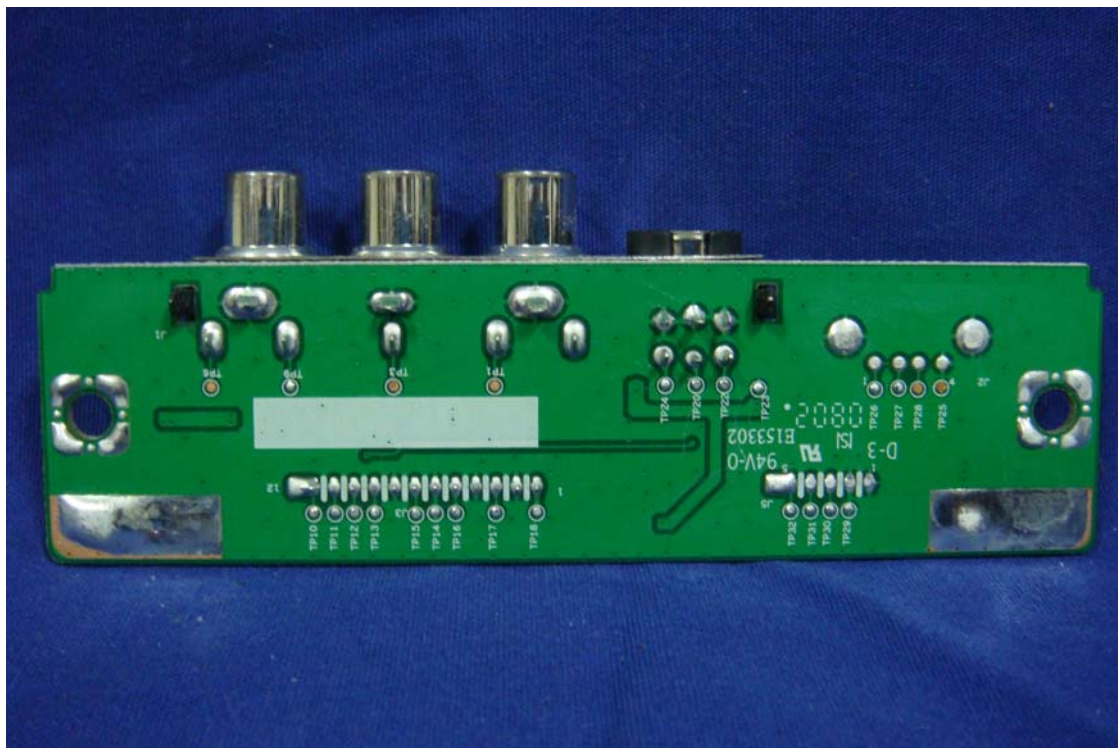
(18) EUT Photo
