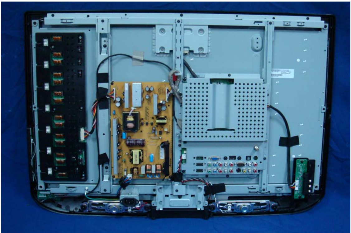
(6) EUT Photo
