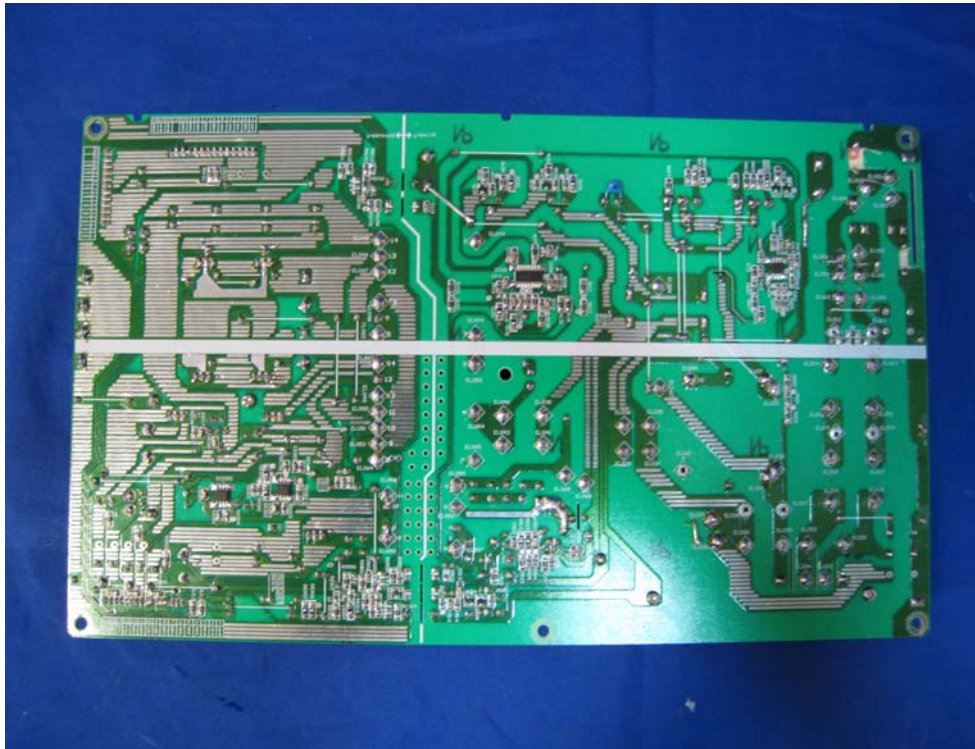
(9) EUT Photo
