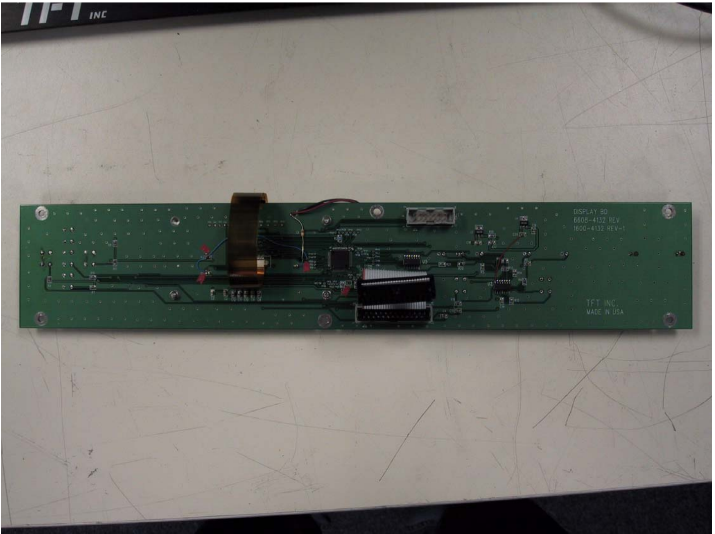
Display PCB – Top
