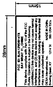
SCALE 2:1
