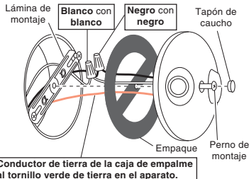
Cableado del reflector
