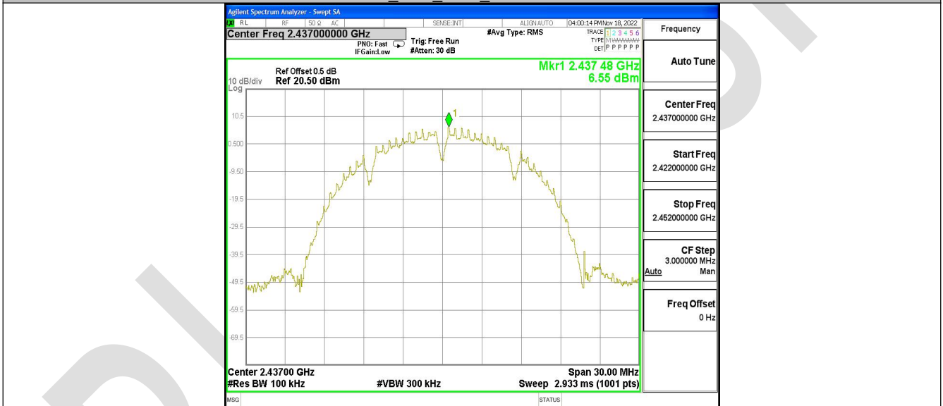
11B_Ant1_2437_0~Reference
