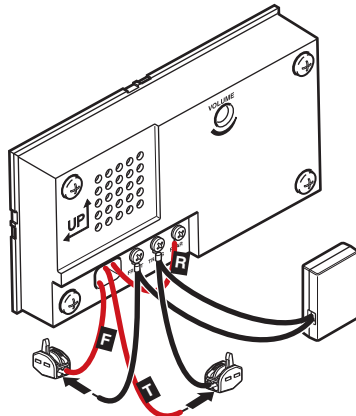
Ejemplo 1: Campana electrónica
