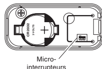
Interrupteur d'entrée
