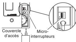
Interrupteur d'appoint
