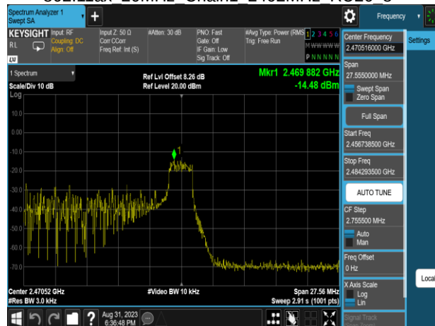
802.11ax 20MHz Chain1 2462MHz RU52 40
