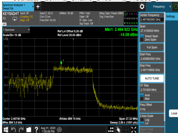
802.11ax 20MHz Chain0 2462MHz RU26_8
