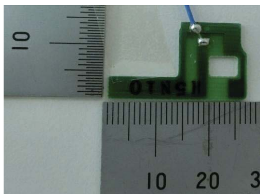
ANT/WIFI/***-KTR
